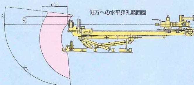
GEOKID TNS-15型 穿孔作業範囲図
